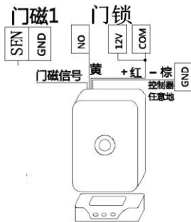
电控锁接线示意图
